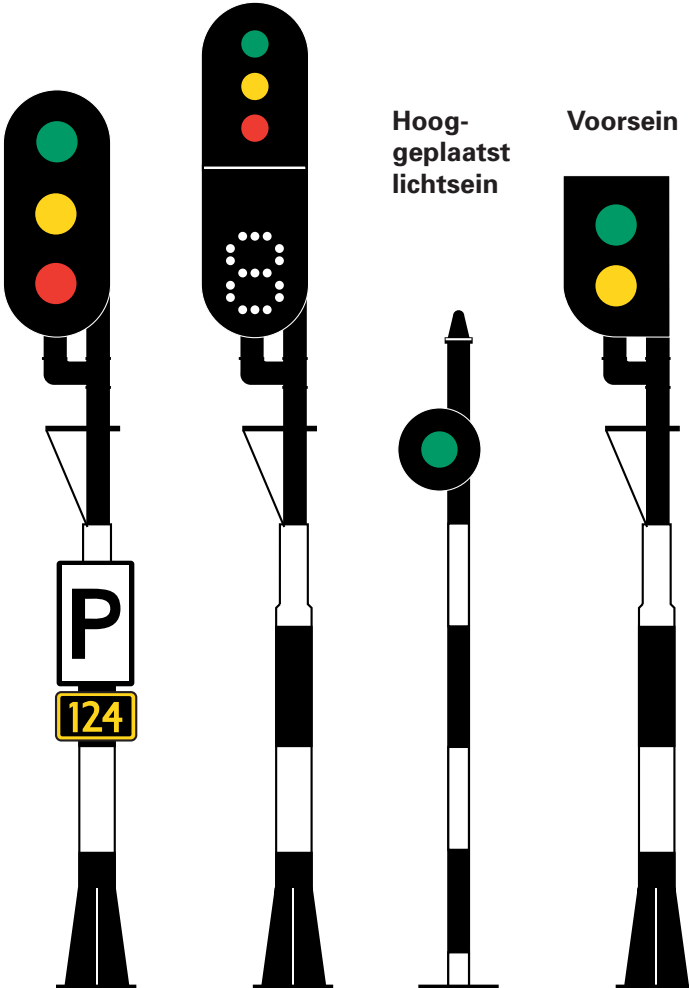
Hooggeplaatst lichtsein met cijferbak
